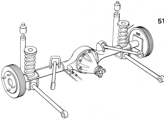
MODEL 510 S.W. ( '69-73)
